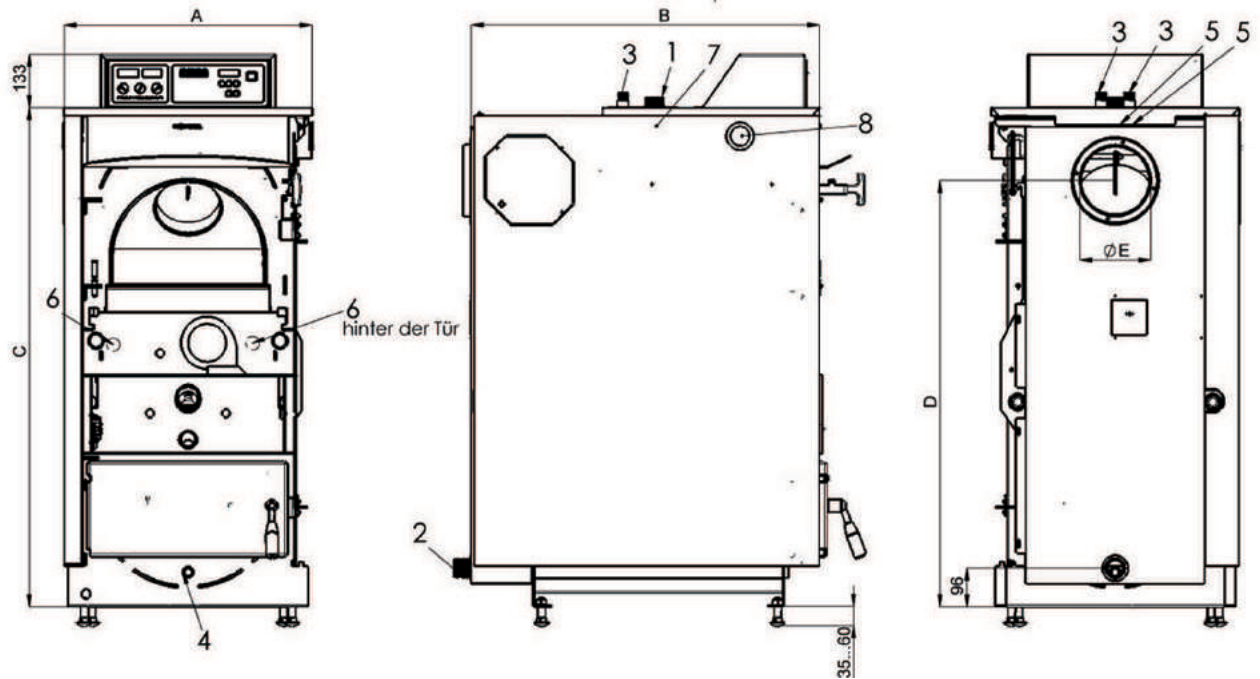
Abbildung 22: Ansicht HV
