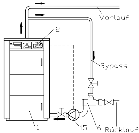
Abbildung 18: Der Kesselkreis
