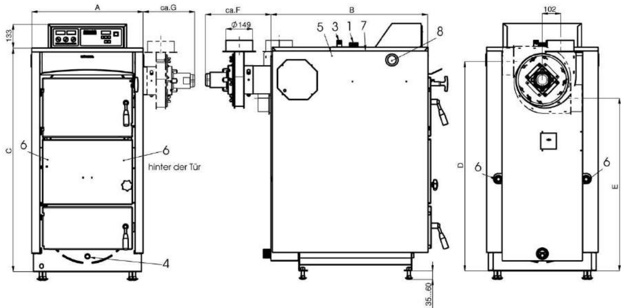
Abbildung 23: Ansicht HV-S
