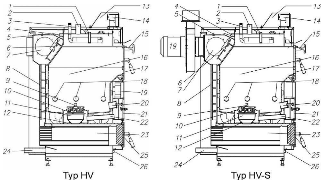
Abbildung 6: Der Holzvergaser-Heizkessel
