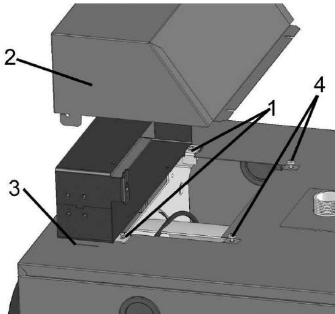
Abbildung 1: Die Schaltfeldmontage
