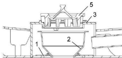
Abbildung 8: Der Turbobrenner im Schnitt
