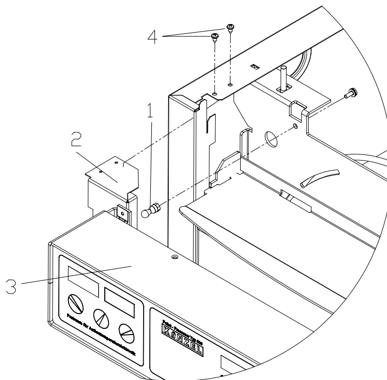
Abbildung 2: Die Schaltfeldmontage Typ HV-RL
