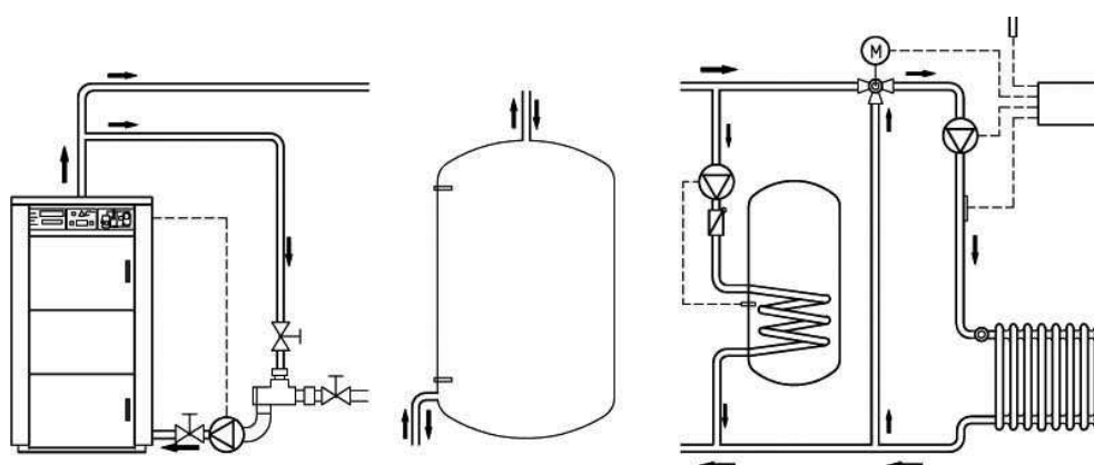
Abbildung 16: Kesselkreis Pufferkreis Verbraucherkreis
