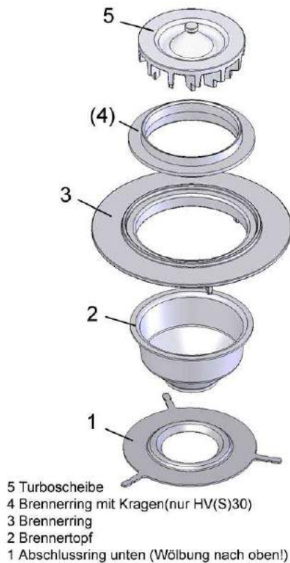
Abbildung 7: Der Turbobrenner
