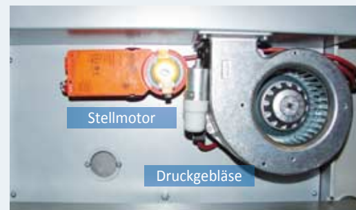
Die optimale Luftmengeneinstellung erfolgt mittels Stellmotor.
