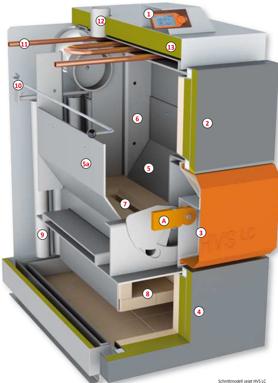
Schnittmodell zeigt HVS LC Technische Änderungen vorbehalten
