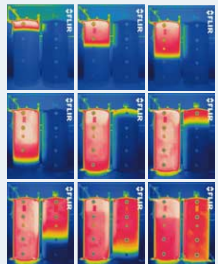
Die hier gezeigte Zeitrafferaufnahme zeigt deutlich erkennbar die gleichmäßige Verteilung und Schichtung der Wärmeenergie bei der Beladung des Speichers.
