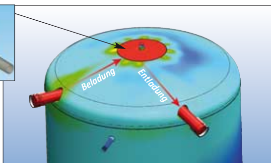
Schichtleitsystem SLS® (oben und unten im Speicher vorhanden)
